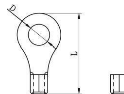
Kroužková svorka:
